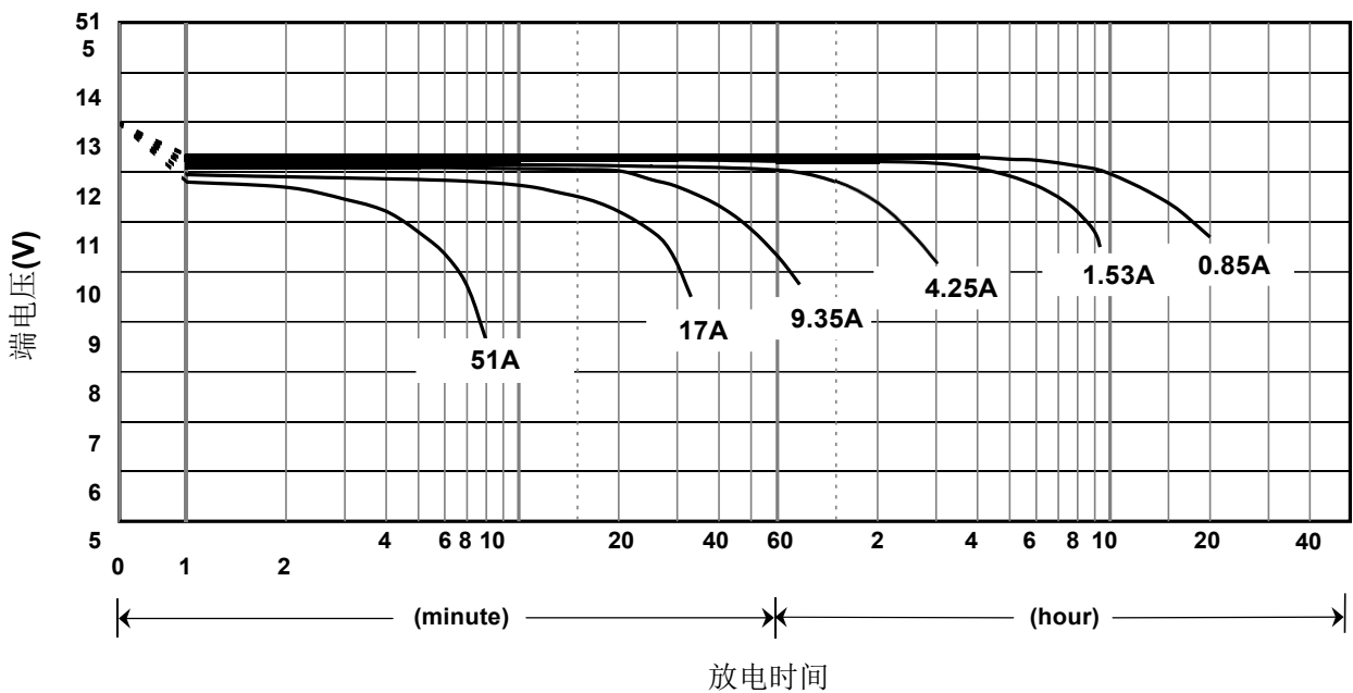
■放电特性(25°C)
